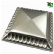
Основание балясины штампованное, арт. 8.880 170x170x1мм Вес: 0.27 кг Цена: 135 руб.
